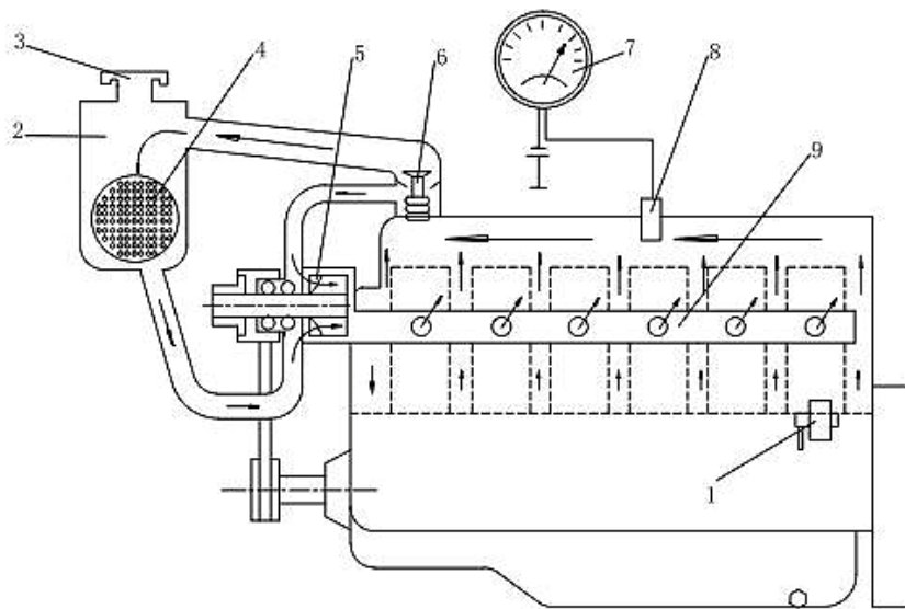
Figura 11: Diagrama de enfriamiento.
