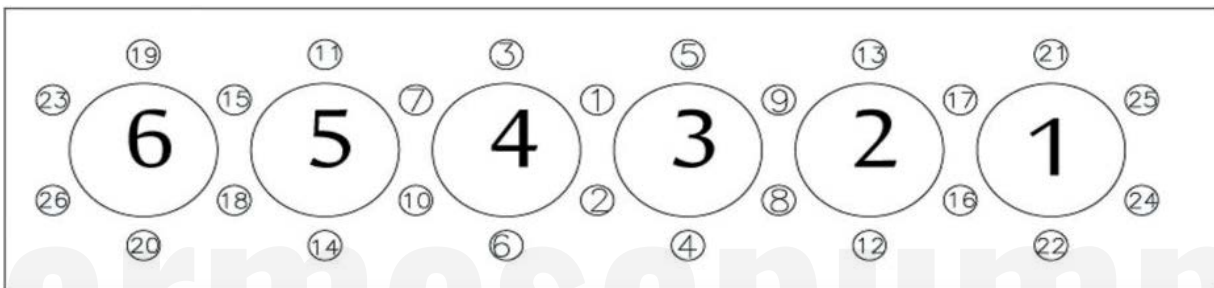
Figura 4: Secuencia de apriete de los pernos en la culata.
