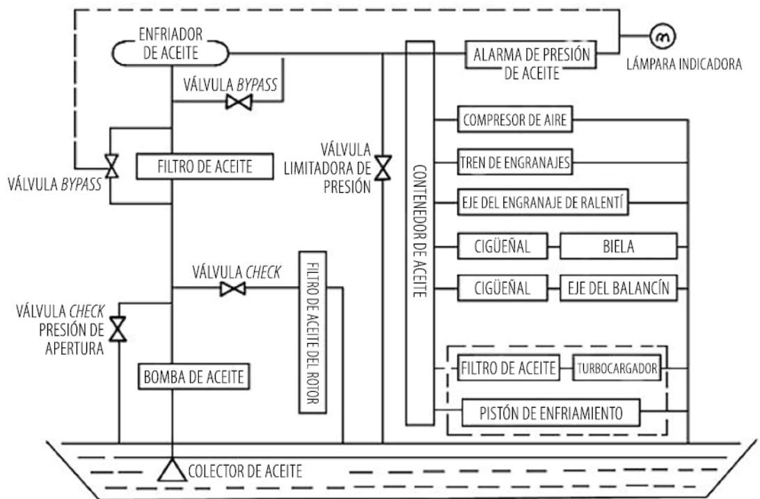
Figura 10: Sistema de lubricación.
