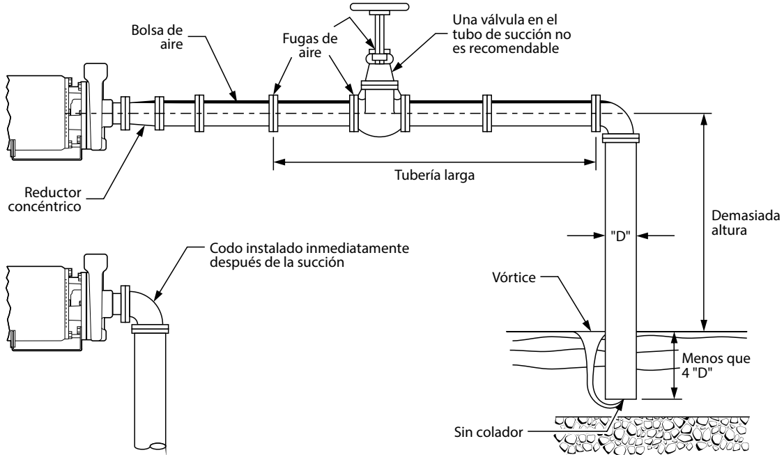
Figura 2 Instalación incorrecta.
